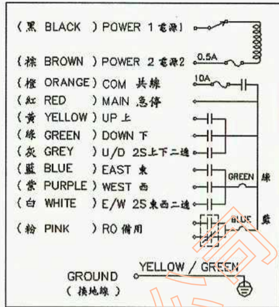
F21-4D 接線圖
