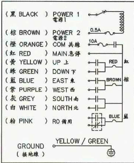
F21-E1/E1B 接線圖
