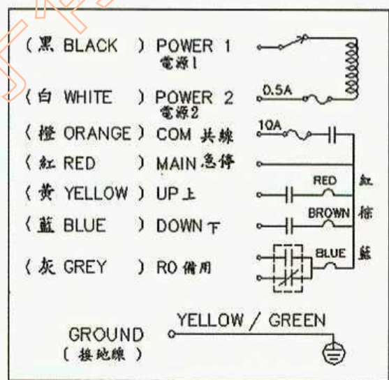
F21-2S 接線圖
